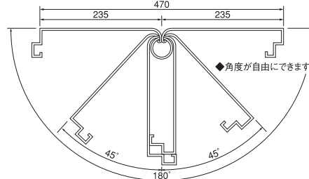
■コーナー用断面図
